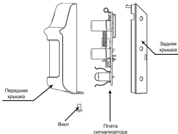
Рис.1 Конструкция сигнализатора
